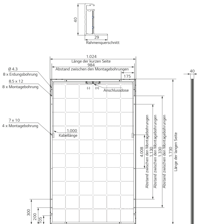
Der Abstand gilt zwischen den Mittelpunkten der Montage- und Erdungsbohrungen.
